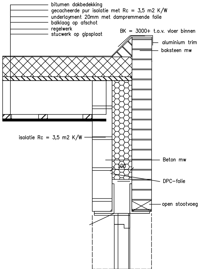
Detail 2 achtergevel
