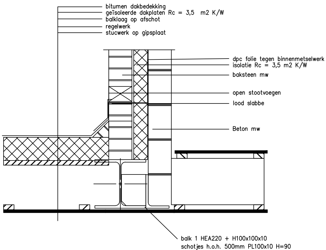
Detail 1: dakdetail aansluiting achtergevel
